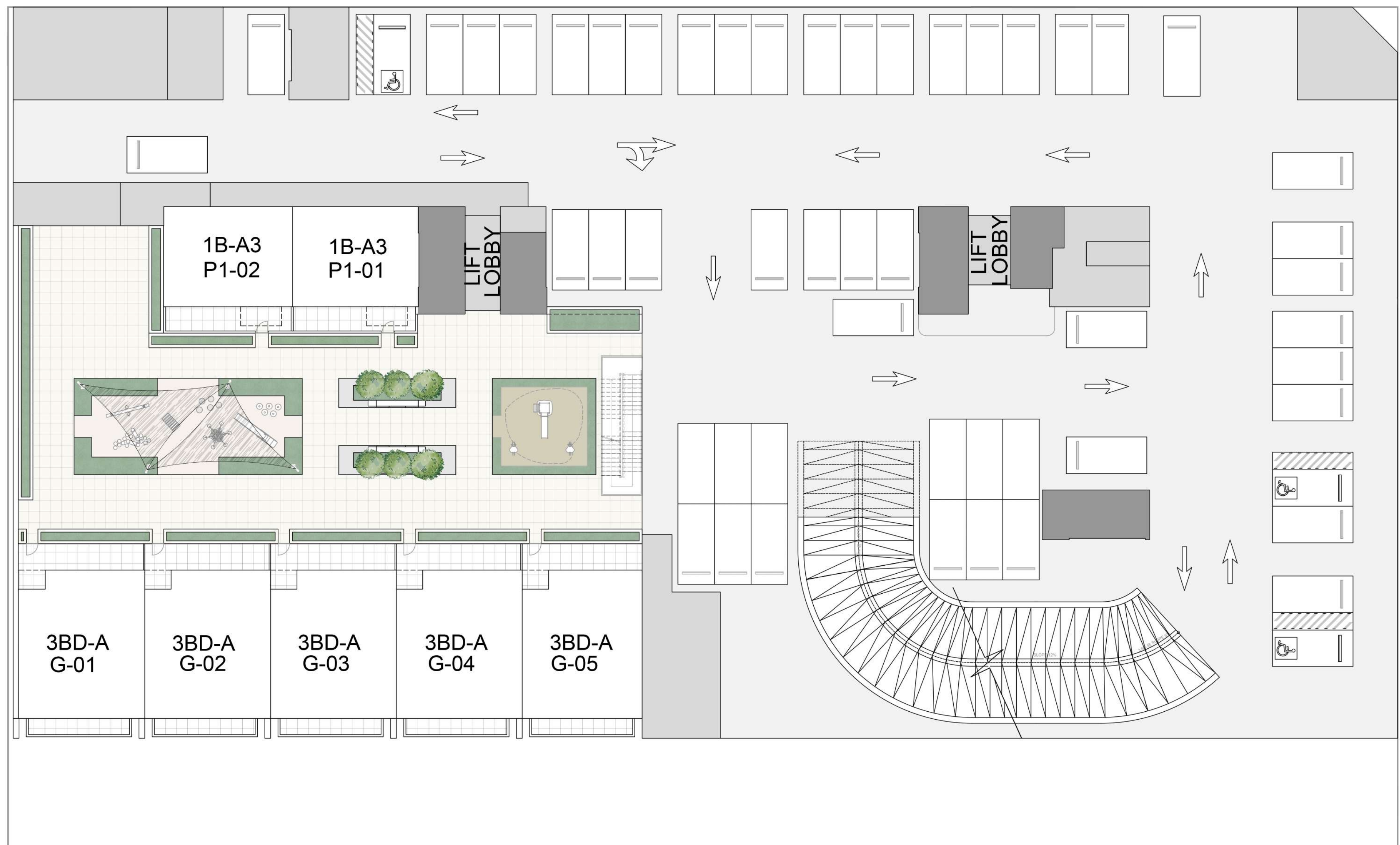
PODIUM 1
