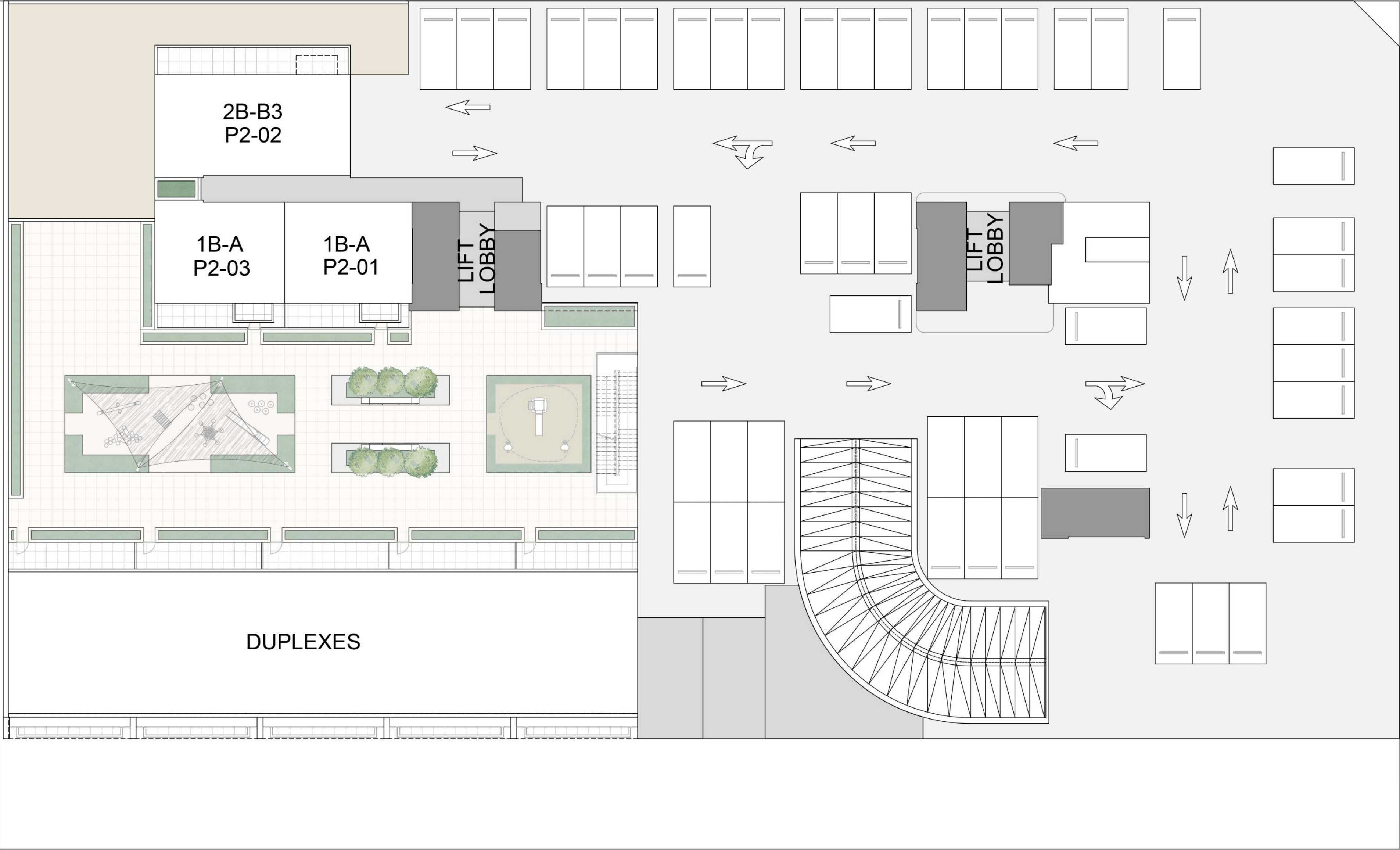
PODIUM 2
